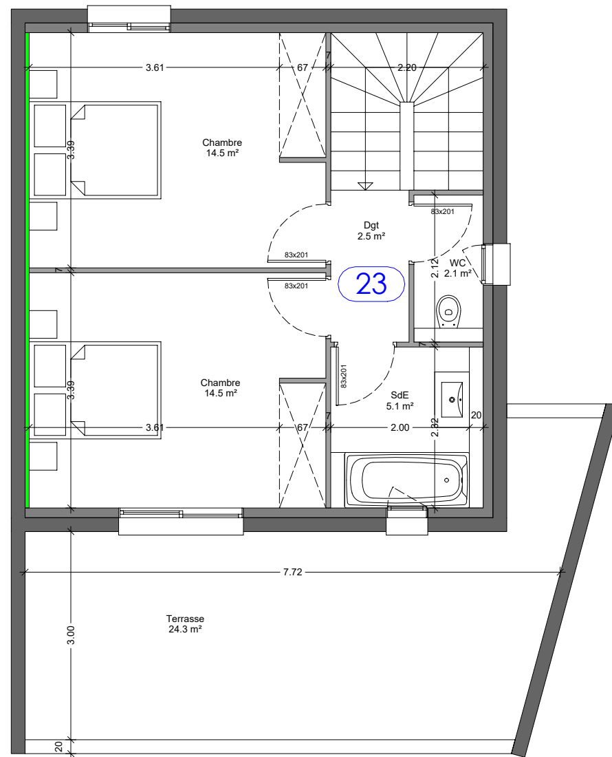
Niveau R+1
