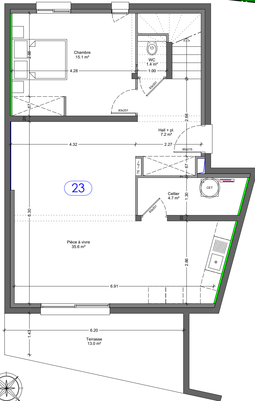
Niveau RdC
