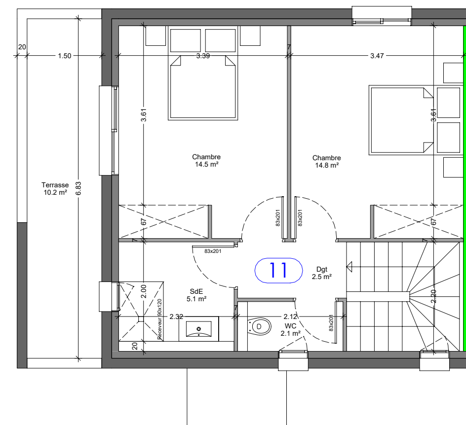
Niveau R+1
