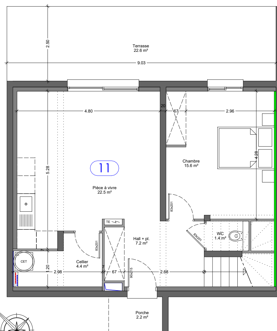
Niveau RdC
