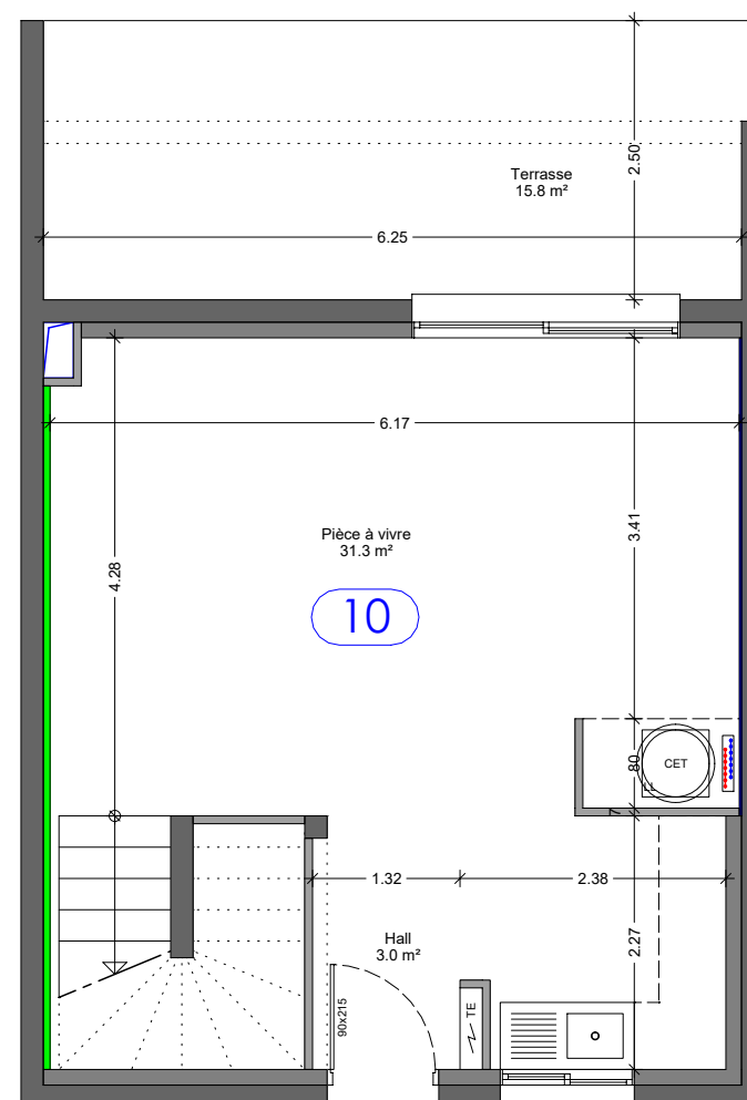
Niveau RdC
