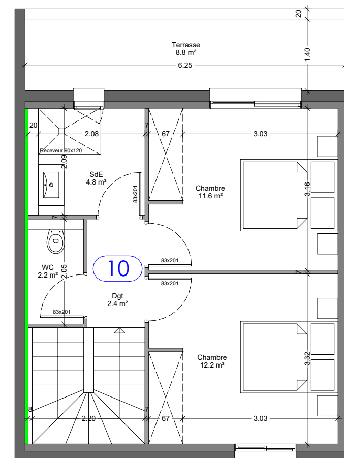
Niveau R+1
