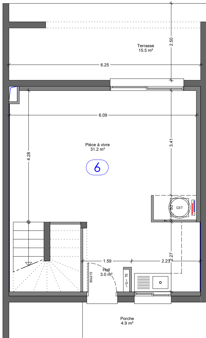
Niveau RdC
