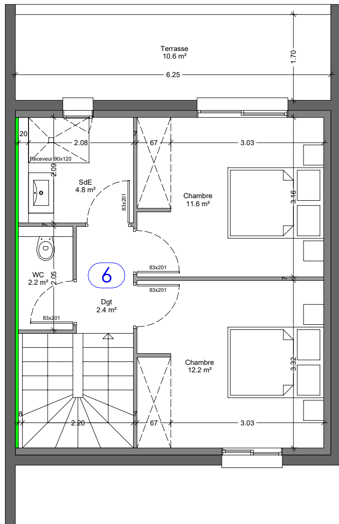
Niveau R+1
