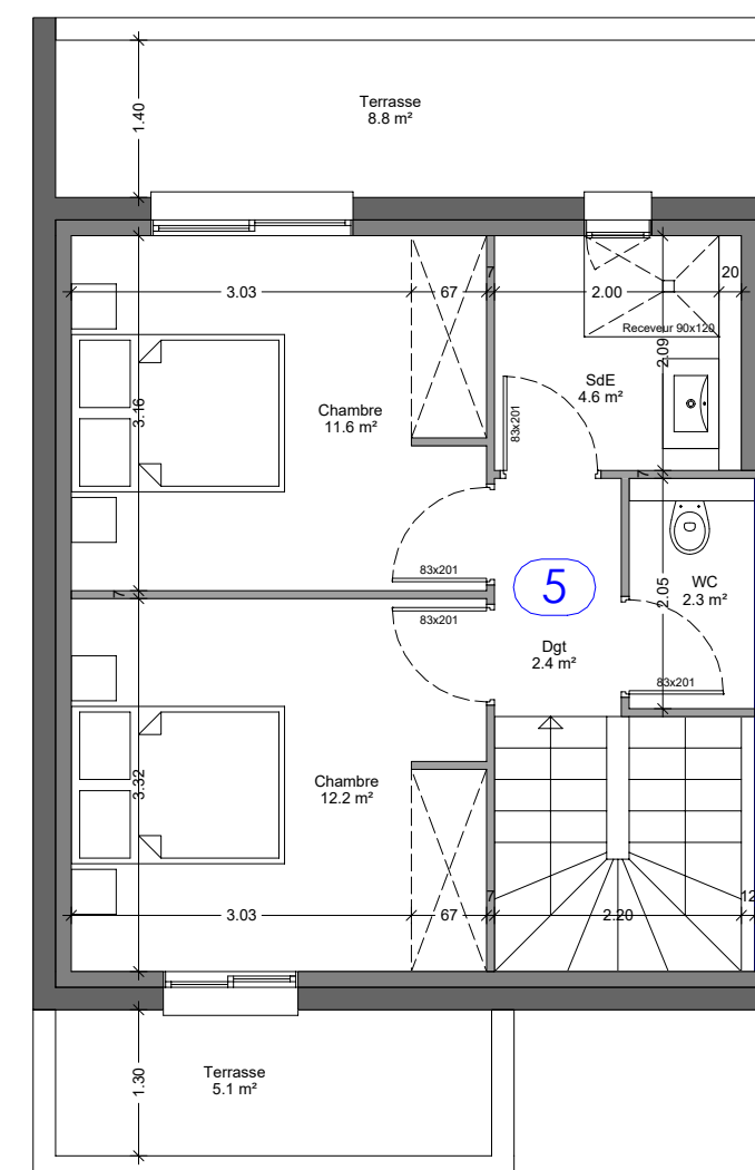
Niveau R+1
