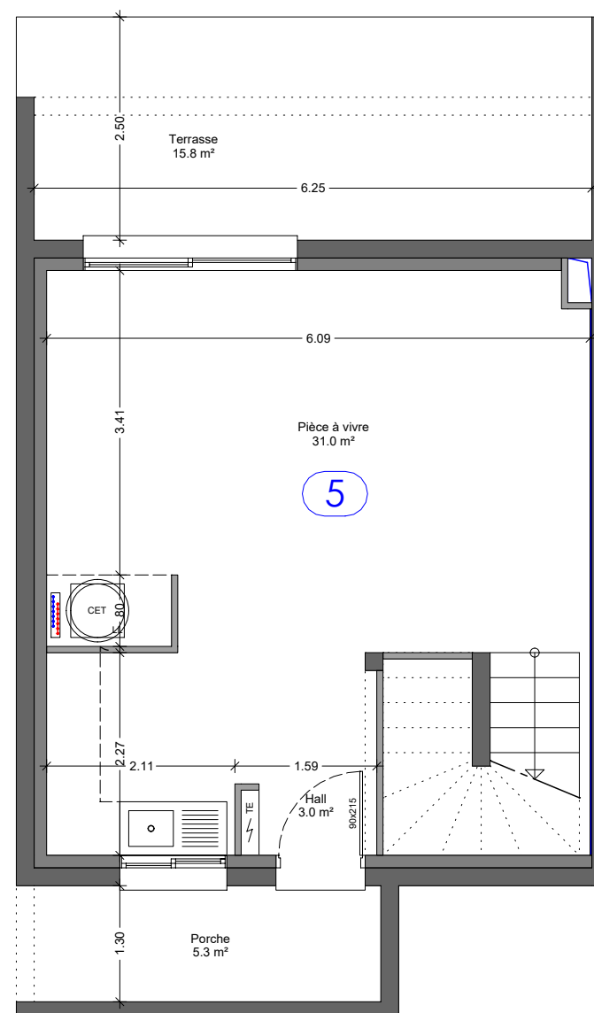
Niveau RdC
