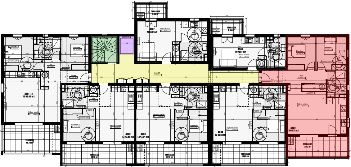
Plan d'étage courant R+3
