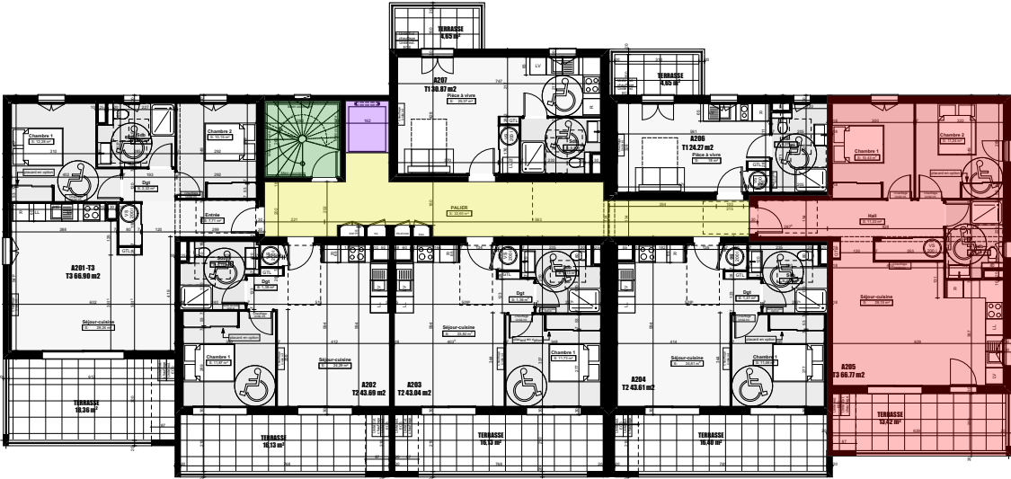
Plan d'étage courant R+2
